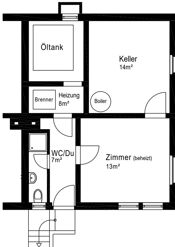
Untergeschoss
